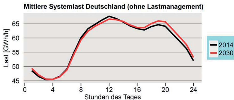
Abbildung 2: Mittlere Systemlast Deutschlands im Vergleich der Jahre 2014 und 2030
