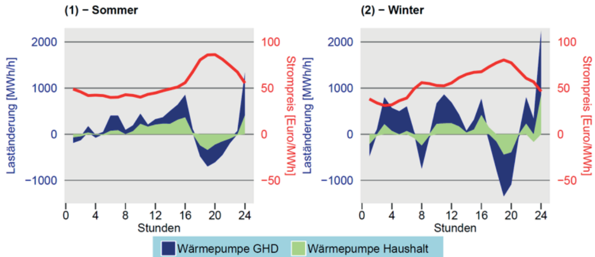
Abbildung 3: Änderung der Wärmepumpenlast vor und nach Lastmanagement sowie mittlerer Strompreis vor Einsatz von Lastmanagement
