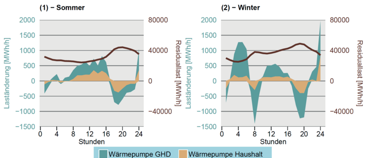
Abbildung 5: Änderung der Wärmepumpenlast unter Nutzung der Residuallast als Preissignal
