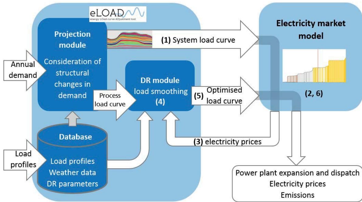
Abbildung 1: Aufbau des gekoppelten Modells
